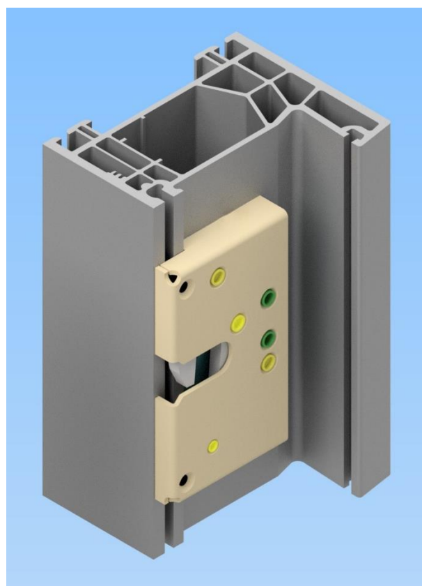
Рисунок 2. Крепление защелки к профилю рамы.
