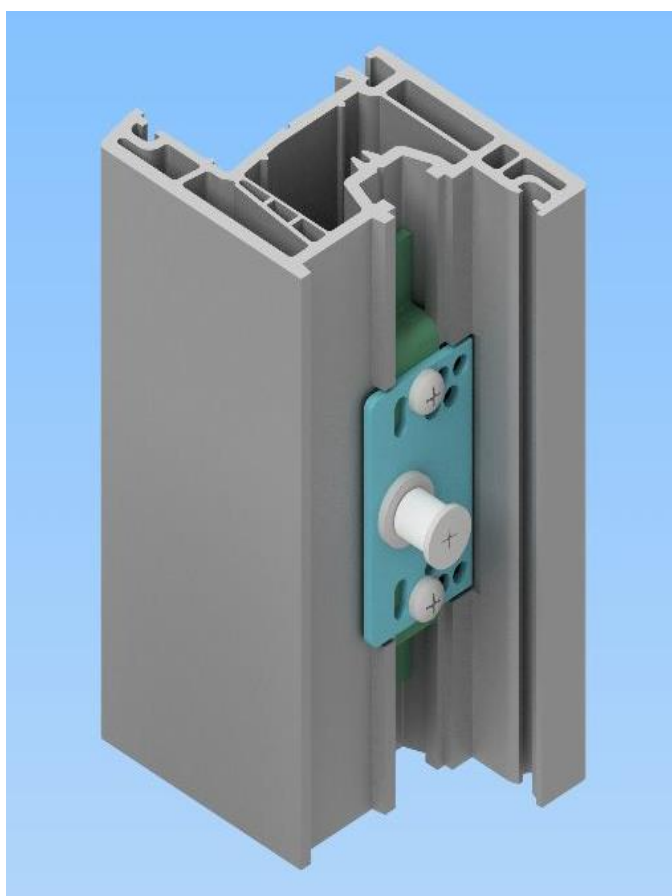
Рисунок 1. Крепление ригеля к профилю створки.
