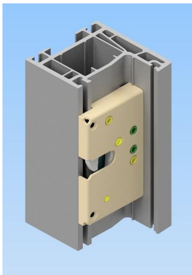
Рисунок 2. Крепление защелки к профилю рамы.
