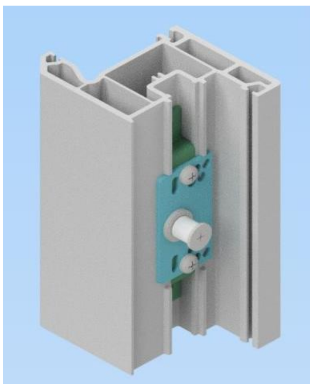
Рисунок 1. Крепление ригеля к профилю створки.
