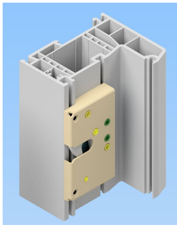
Рисунок 2. Крепление защёлки к профилю рамы.
