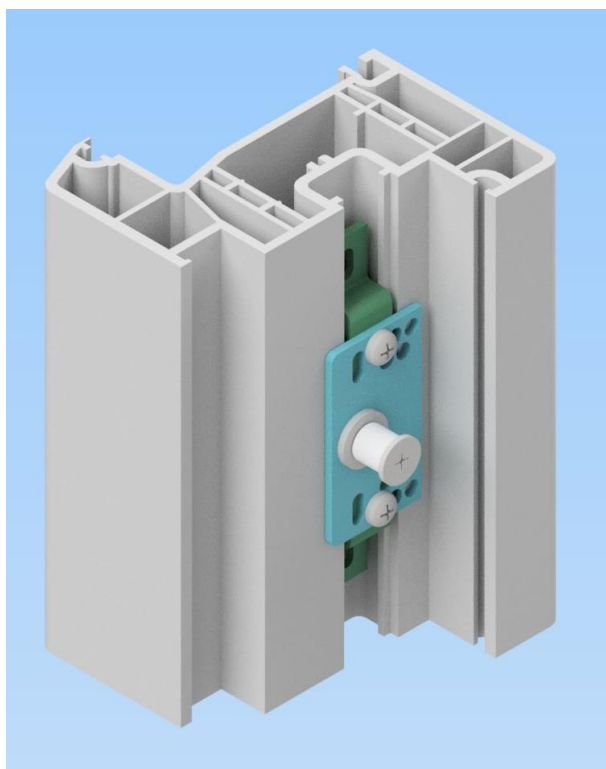
Рисунок 1. Крепление ригеля к профилю створки.
