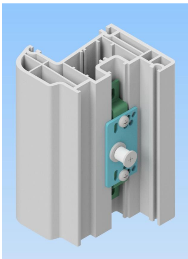
Рисунок 1. Крепление ригеля к профилю створки.
