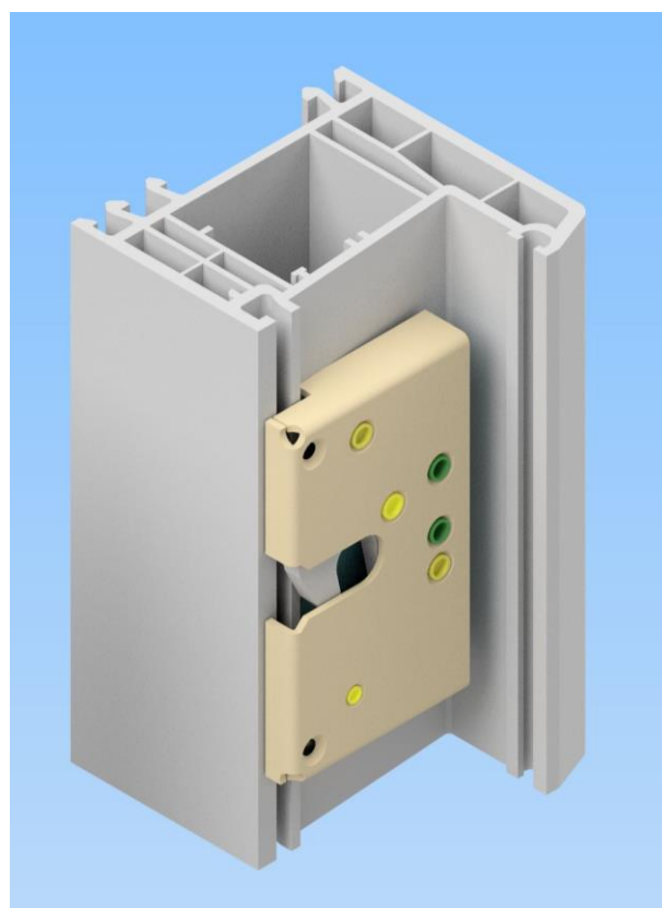
Рисунок 2. Крепление защёлки к профилю рамы.
