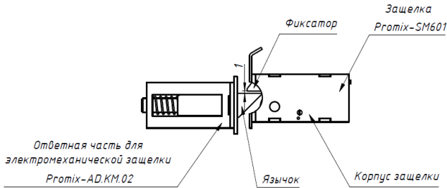
Рис. 3 Взаимное расположение защелки и ответной части при установке
