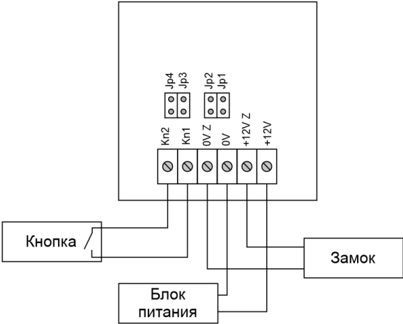
Рис. 1 Схема подключения
