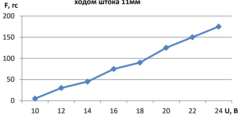
График зависимости втягивающего усилия от напряжения с ходом штока 11мм
