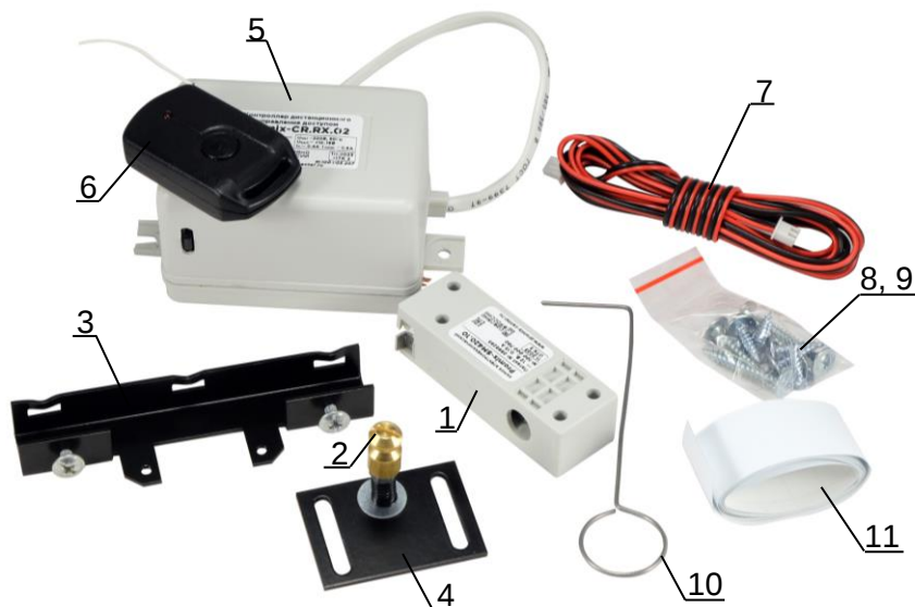
Рис.2. Комплект Promix-FRS.1D.04
