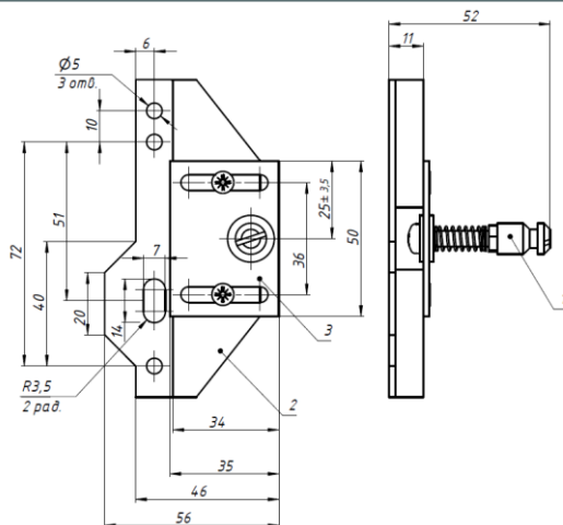
Рис. 4. Габаритные и установочные размеры ригеля Promix-AD.DB.16 поз. 1 в сборе с кронштейнами Promix-AD.BR.16 поз. 2, Promix-AD.BR.18 поз. 3
