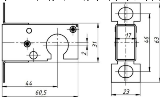
Рис.3 Габаритные размеры
