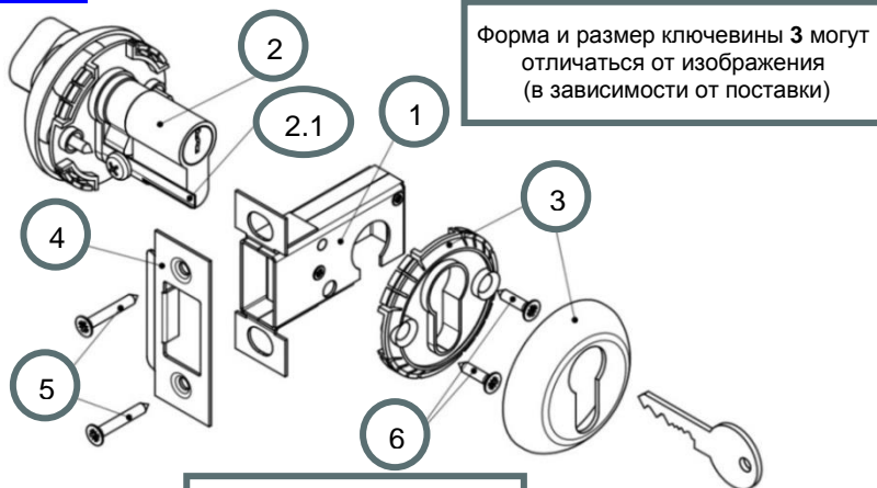
Рис.2 Конструкция механизма
