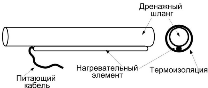
Рис.2. Монтаж обогревателя
