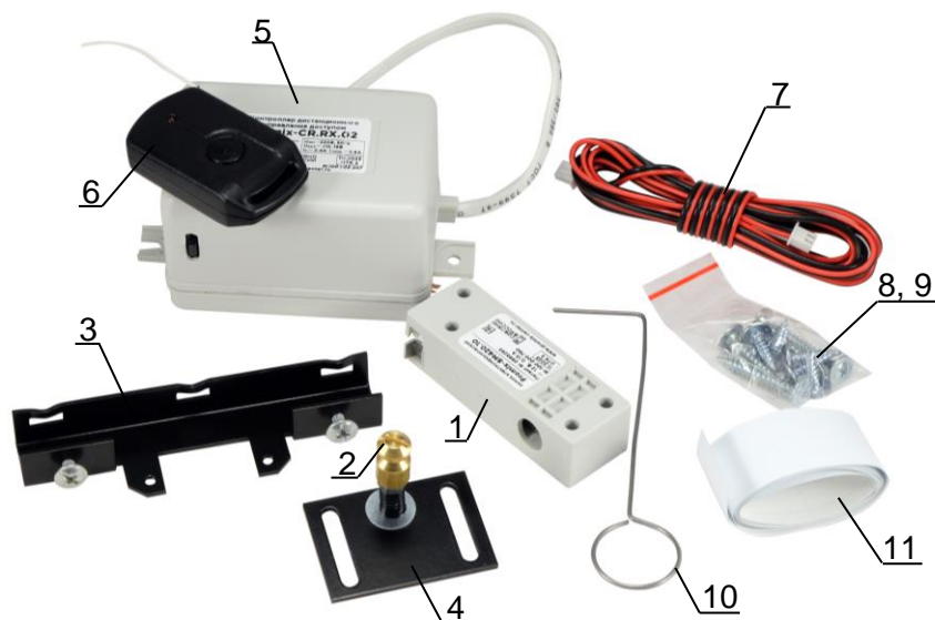
Рис.2. Комплект Promix-FRS.1D.04
