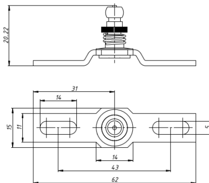
Рис. 3. Ригель Promix-AD.DB.12
