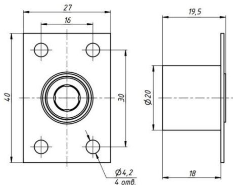
Рис. 2. Замок Promix-SM131.10
