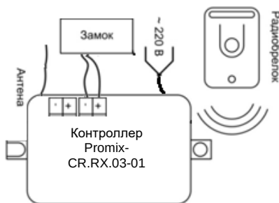
Рис.1.Блок-схема подключения комплекта
