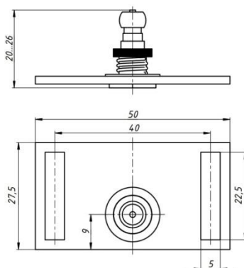
Рис. 3. Ригель Promix-AD.DB.13
