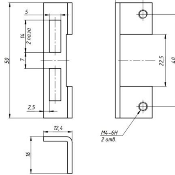
Рис. 5. Кронштейн Promix-AD.BR.06
