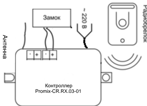
Рис. 16. Схема подключения контроллера
