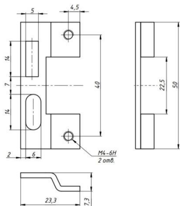
Рис. 4. Кронштейн Promix-AD.BR.05
