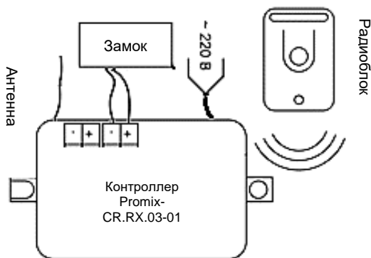
Рис.1.Блок-схема подключения комплекта
