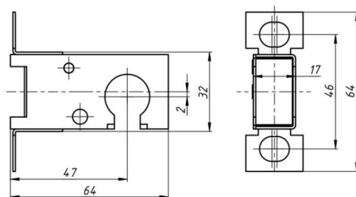
Рис.3 Габаритные размеры
