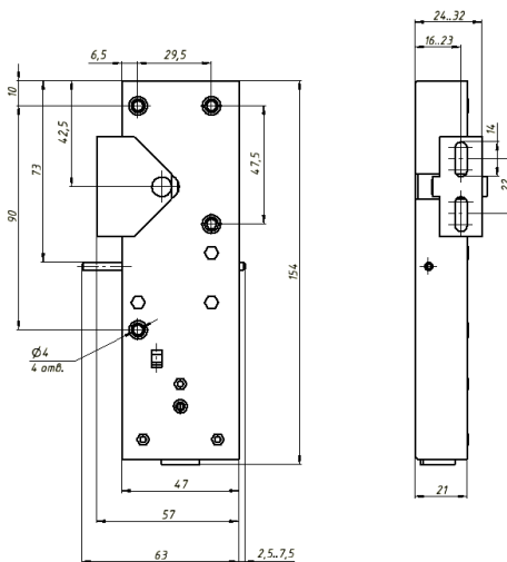
Рис. 4. Монтаж замка и ригеля.
