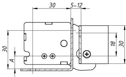
Рис. 3. Взаимное расположение для замка и ригеля модификаций: Promix-SM330 TC.10.2, Promix-SM330.10.2, Promix-SM330.10.2-01, Promix-SM330.10.3, Promix-SM330.10.3-01, Promix-SM330.11.2, Promix-SM330.11.2-01, Promix-SM330.11.3, Promix-SM330.11.3-01
