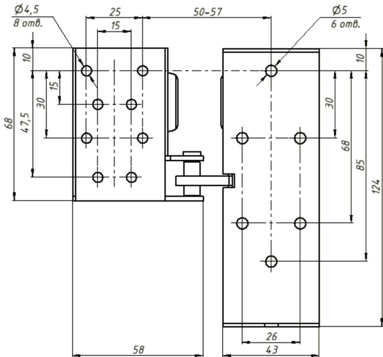
Рис. 4. Габаритные и установочные размеры модификации Promix-SM330.10.3-02 и Promix-SM330.11.3-02
