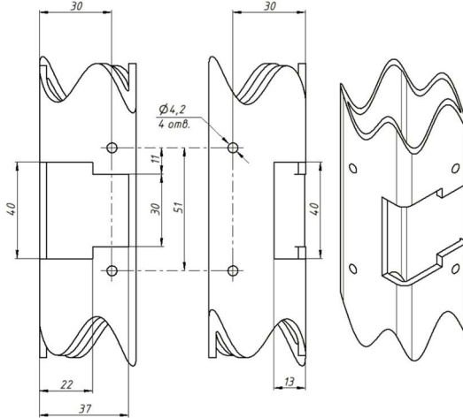
Рис. 1. Размеры необходимых вырезов и расположение отверстий модификаций Promix-SM330.10.2 и Promix-SM330.11.2
