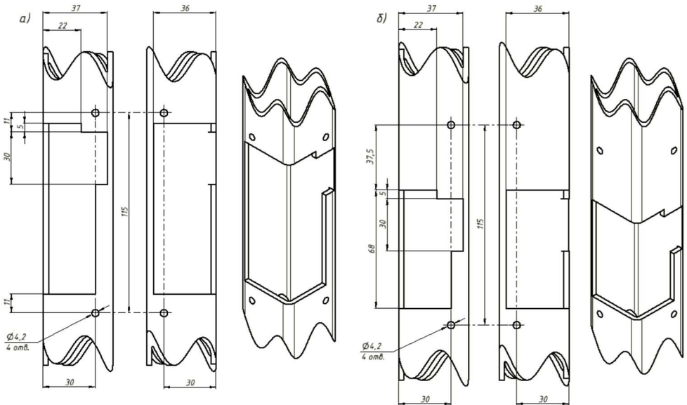
Рис. 2. Размеры необходимых вырезов и расположение отверстий модификаций:
